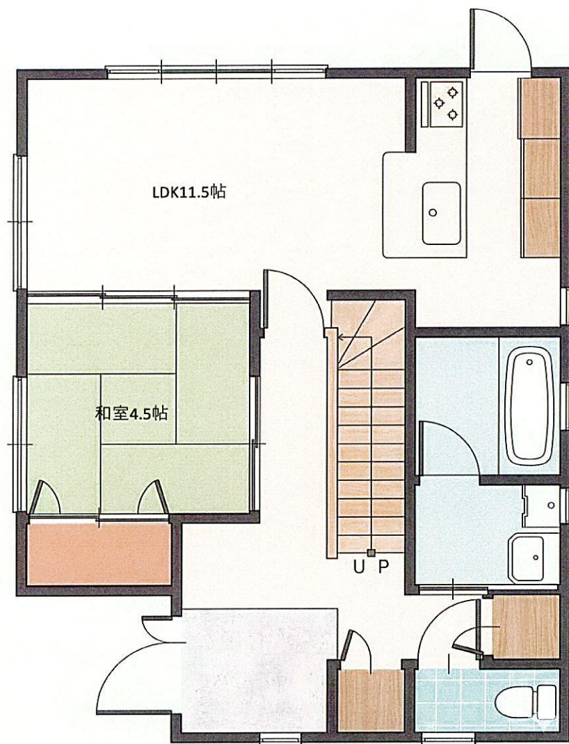
1階
